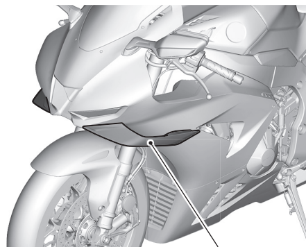
WINGLET (CFRP)
